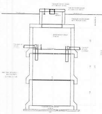
FOSSA SÉPTICA - CORTE
