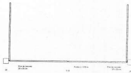
PORTÃO - PLANTA
