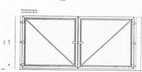
PORTÃO - VISTA FRONTAL
