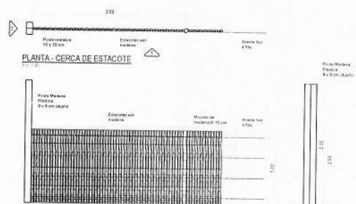
PLANTA - CERCA DE ESTACOTE
