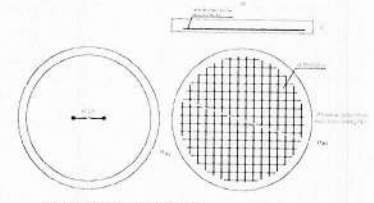
TAMPA DA CAIXA DE INSPEÇÃO
