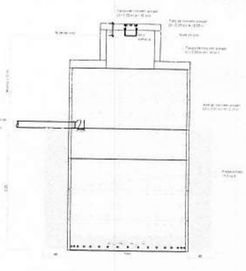
SUMIDOURO - CORTE
