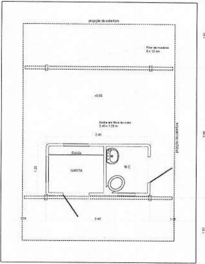
PLANTA
