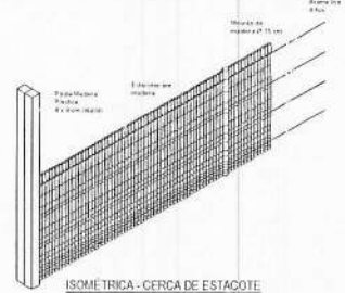
ISOMETRICA - CERCA DE ESTACOTE
