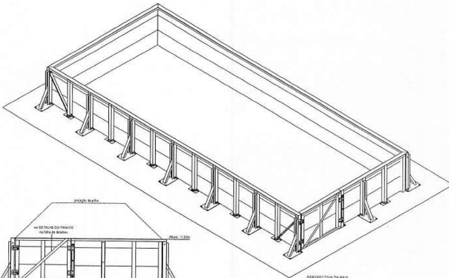
PERPECTIVA DA BAIA
